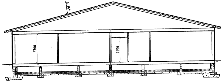
SEKTION B-B
