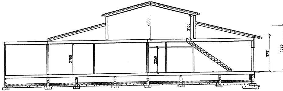
SEKTION A-A
