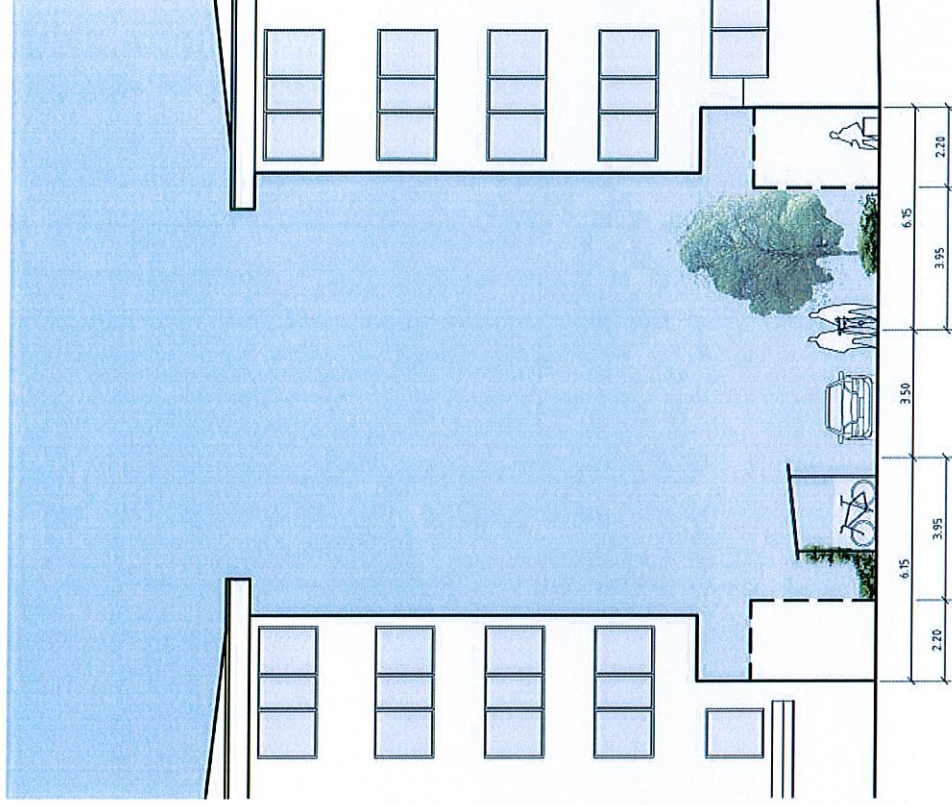
Sektion genom gårdsgatan skala 1:200
