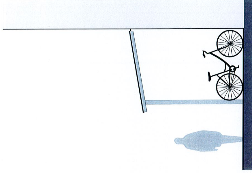
Sektion cykelparkering under tak längs med fasad skala 1:50
