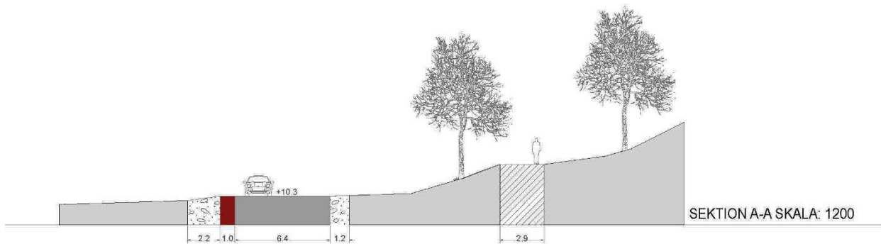
Figur 2a. Principsektion för Hålludsvägens breddning
