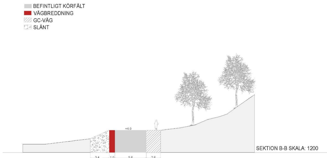
Figur 2b. Principsektion för Hålluddsvägens breddning.
