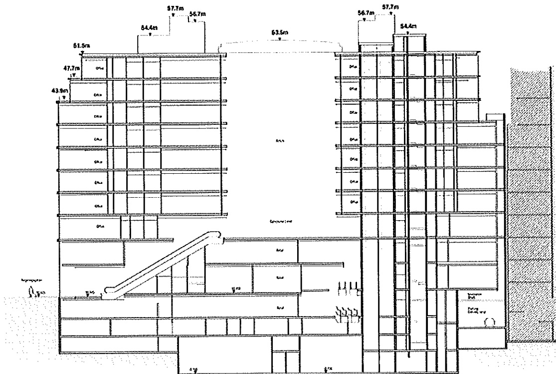
Sektioner genom ny byggnad. Volymstudie av den nya byggnaden ej skalenlig. (SHL Architects) Överst - Tvärsektion genom ny byggnad som visar bostadsdelen mot Mäster Samuelsgatan (till höger i bild). Nederst - Längdsektion.
