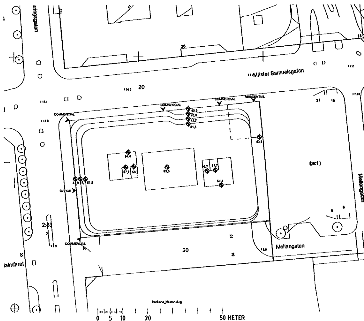
Situationsplan (ej skalenlig) med planerade entrélägen. (SHL Architects)
