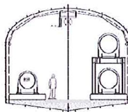
Mätarpassagen
