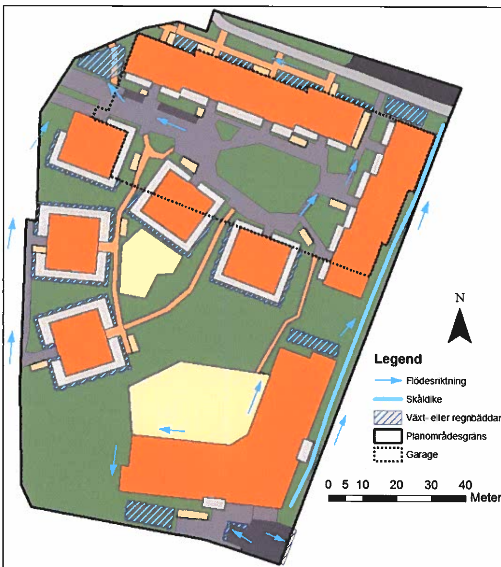
Figur 5-6. Principskiss med förslag till ungefärlig placering av föreslagna anläggningar för dagvattenhantering. Utritade areor är endast exempel och motsvarar inte erforderliga areor.
