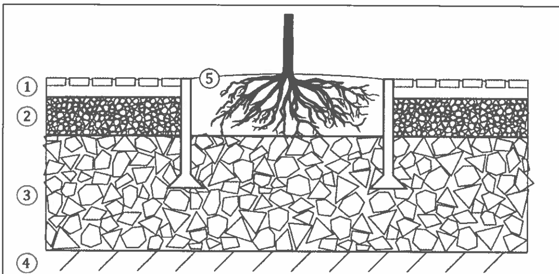
Figur 5-3. Principskiss på en överbyggnad med skelettjord. 1, slitlager 2, luftigt bärlager, 3 skelettjord 4, befintligt luckrad terrass 5, planteringsgrop med växtjord. Illustration Andréa Olsson (2014-06-19)
