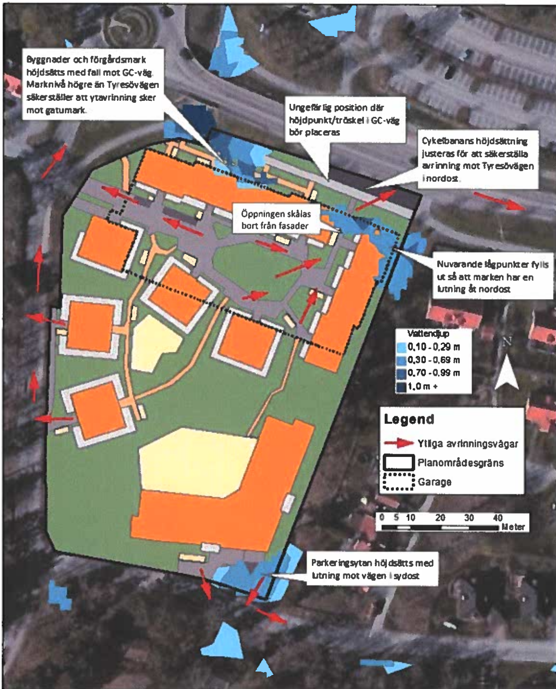
Figur 5-7. Översiktskarta som tar upp några av de aspekter som måste tas i beaktande vid höjdsättning av området för att översvämningsskador ska undvikas.
