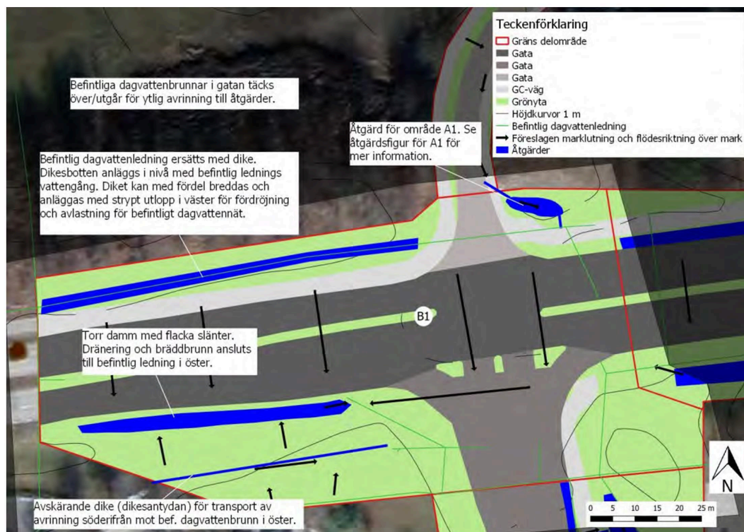
Figur 14. Övergripande dagvattenhantering med föreslagna åtgärder för fördröjning och rening inom delområdet B1. Observera att platser och ytor är ungefärliga och utritade i illustrativt syfte. Bakgrund från Google (Google maps, u.å.).
