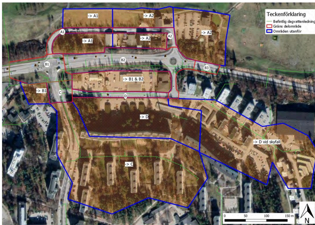
Figur 11. Ytor varifrån flöden transporteras in till utredningsområdet.
