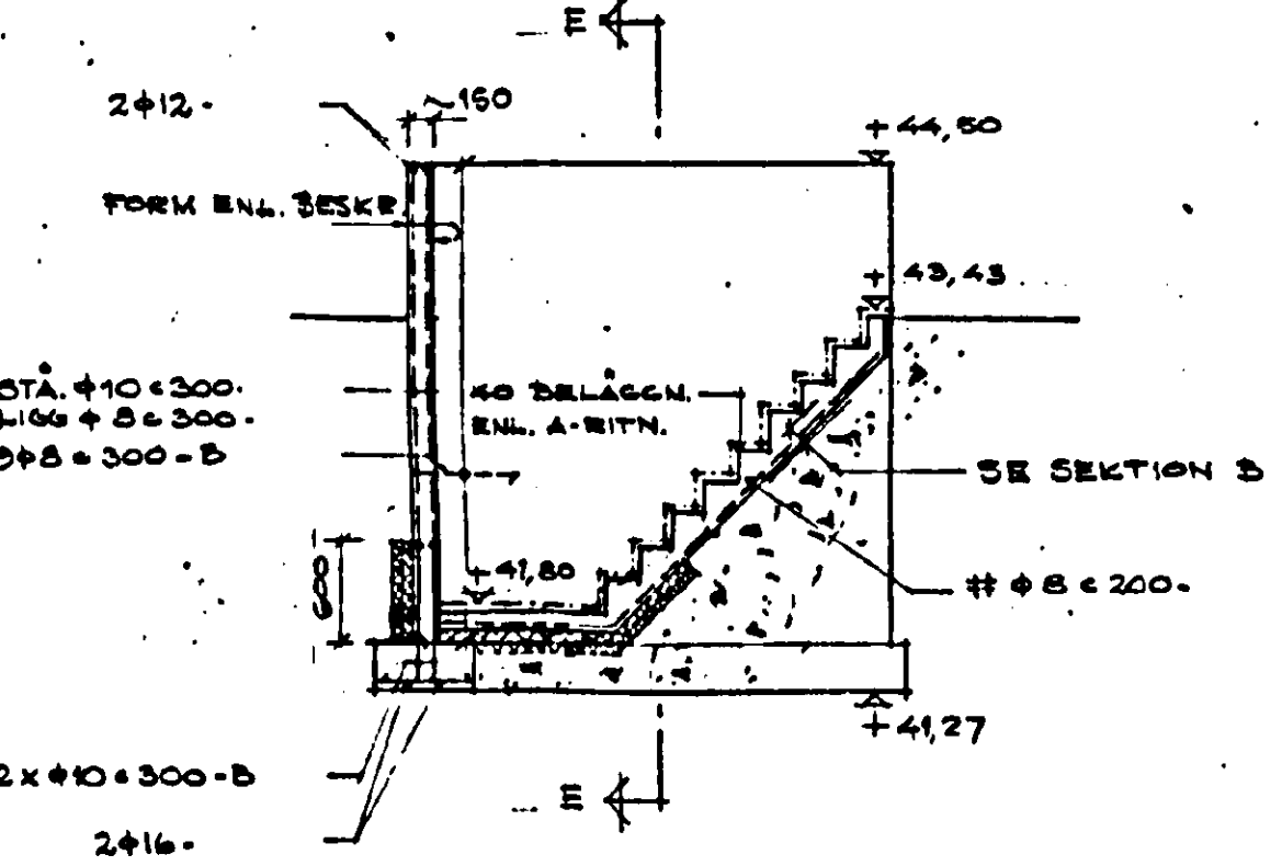
SEKTION D, 1:50 HUS M, TRAPPA E
