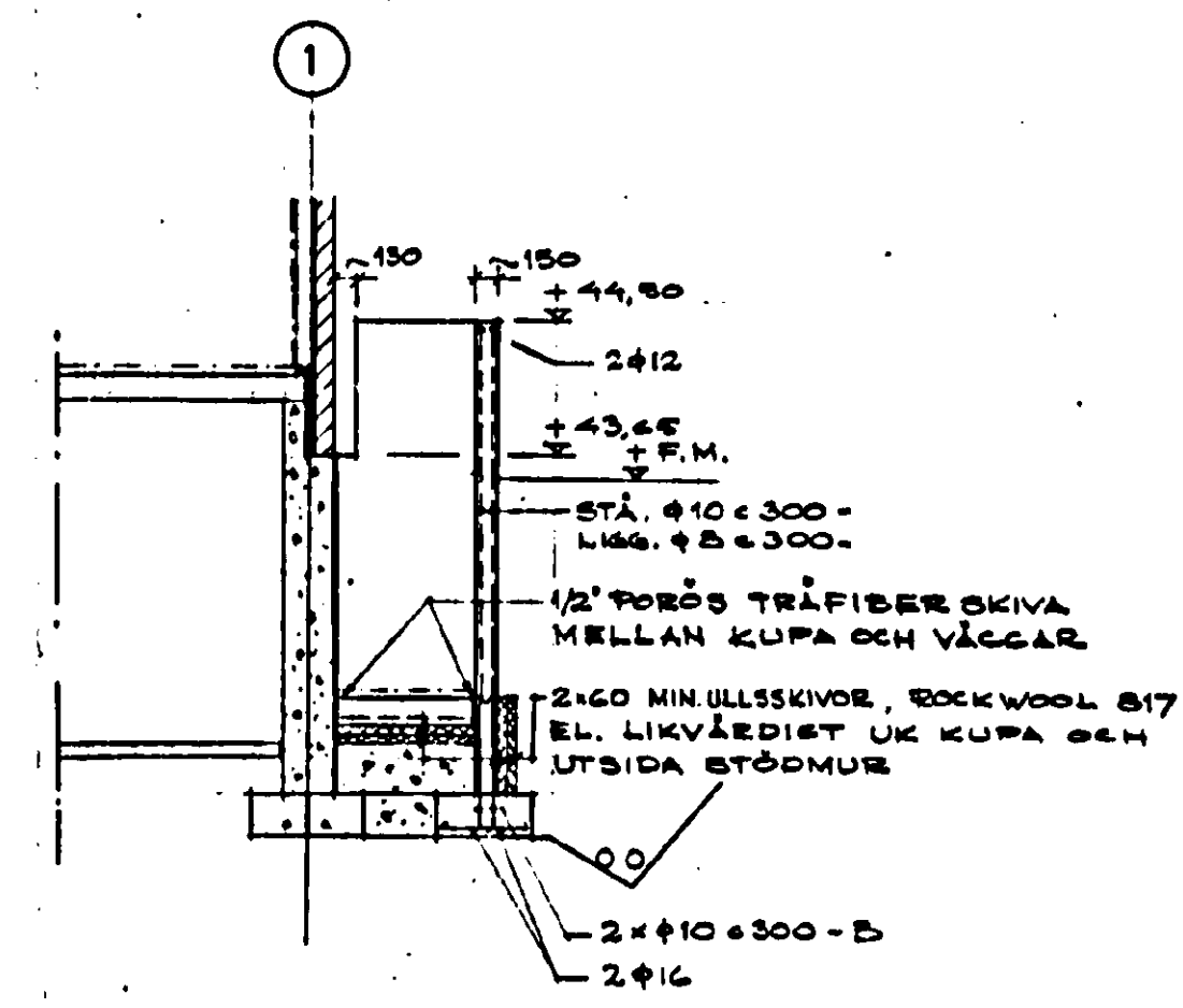
SEKTION E, 1:50
