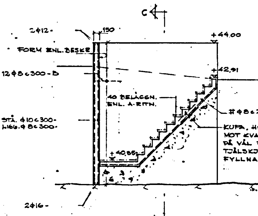
SEKTION B, 1:50 HUS K, TRAPPA D
