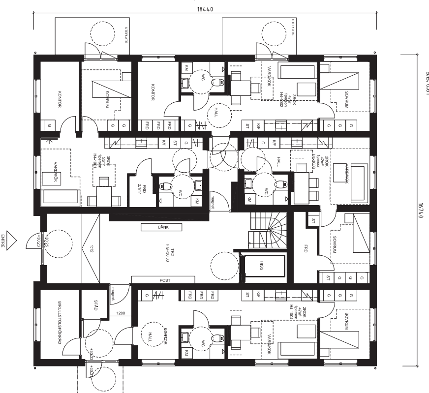
PLAN 10 ENTREPLAN
