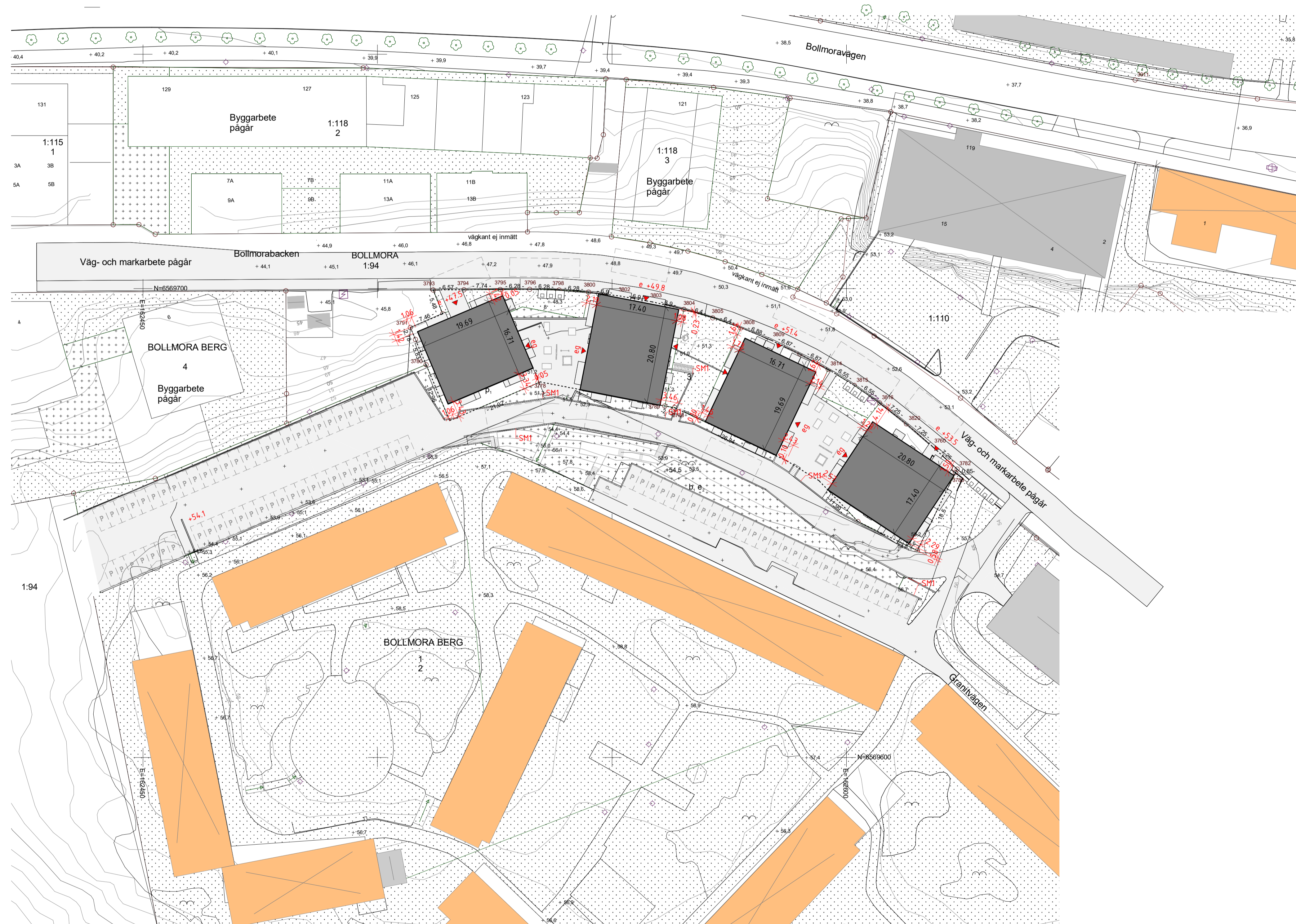
Situationsplan med nybyggnadskarta 1 : 500
