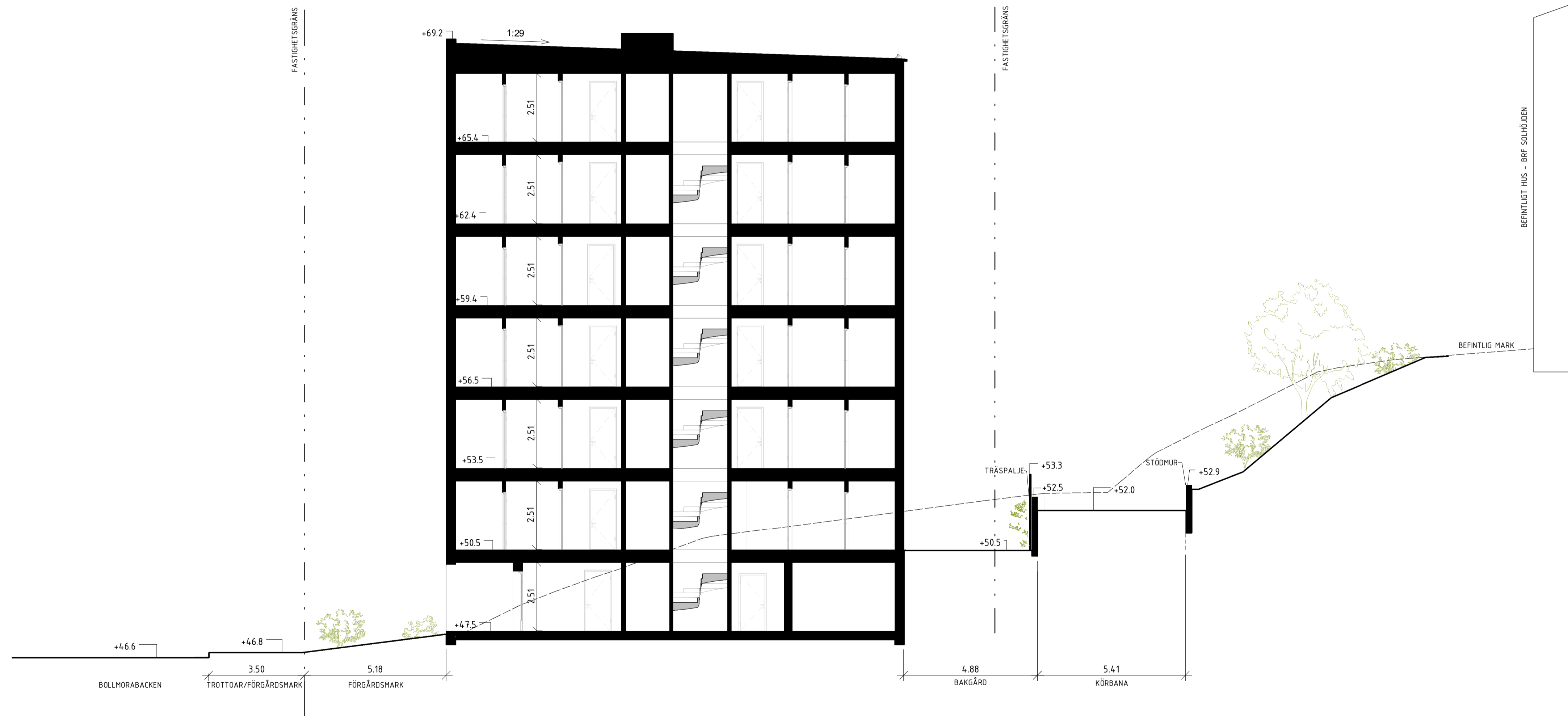
SEKTION A - A 1 : 100
