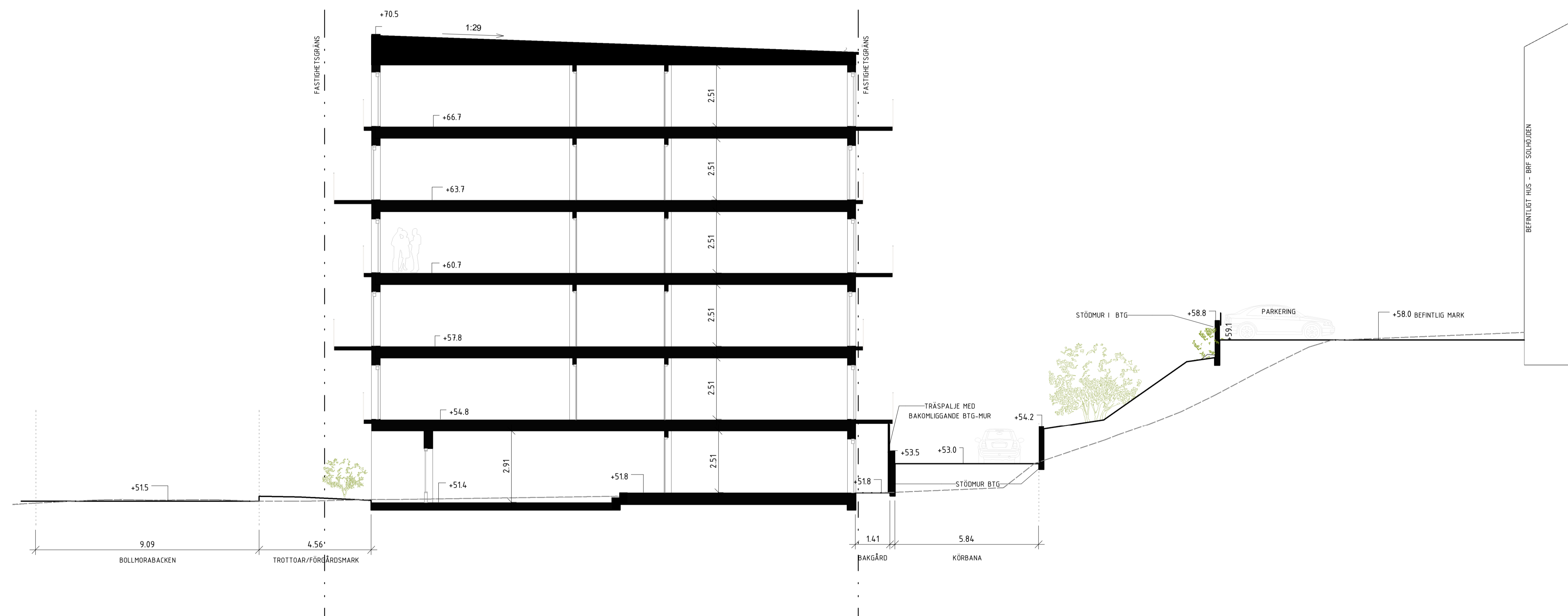
SEKTION C - C 1 : 100
