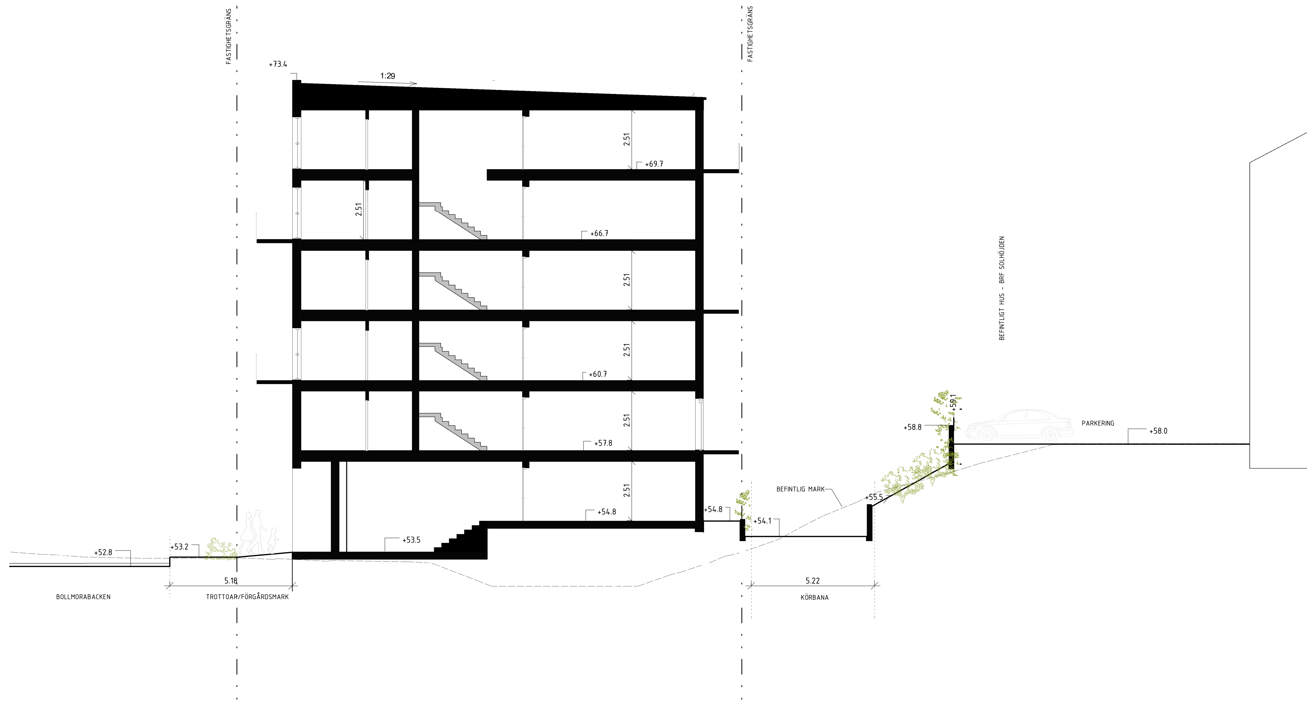
SEKTION D - D 1 : 100
