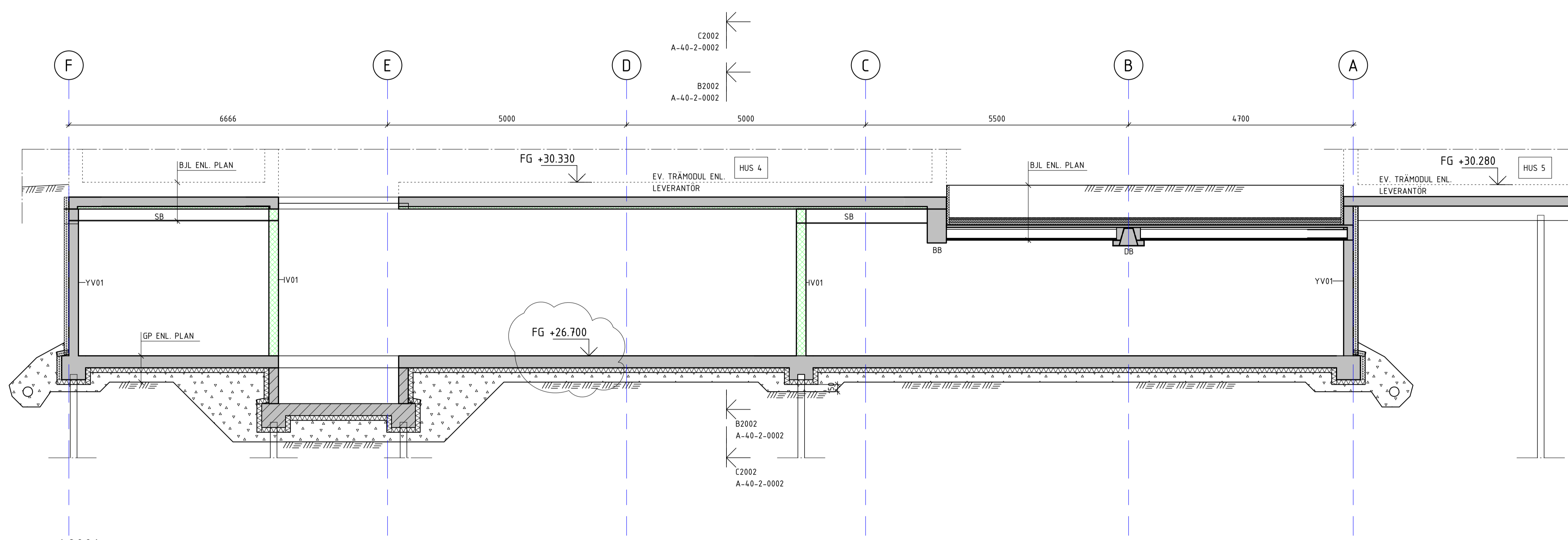
A2001 1 : 50 SEKTION GENOM KORTSIDA
