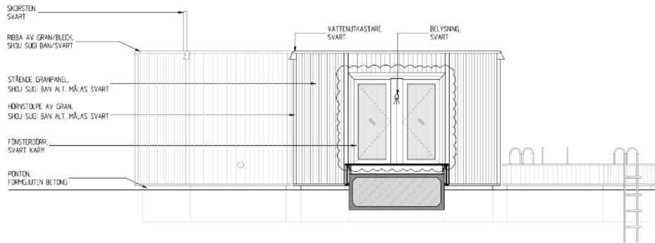
Bild 5. Fasadritning nordost.
