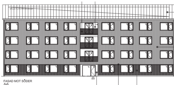
Bild 9. Fasadritning bus 5.
