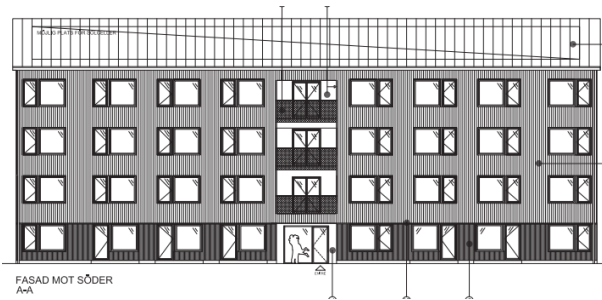
Bild 5. Fasadritning bus 2.
