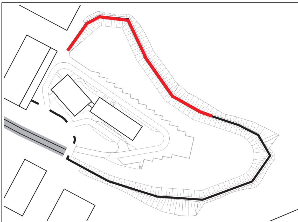
Figur 7. Vid tjock röd linje har bullerskyddsskärmen höjts till 3 m (från 2 m). Övriga bullerskyddsskärmar (tjock svart linje) har befintlig höjd.
