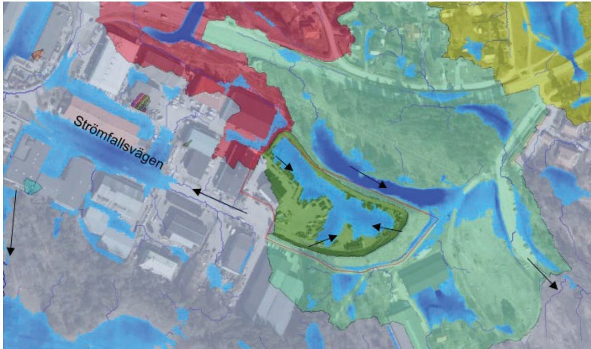
Figur 14. Bild som visar avrinning vid skyfall, samt instängda områden, utan hänsyn till dagvattenledningsnätet. Svarta pilar visar flödesriktning. Utredningsområdet är markerat med röd linje (Bjerkäng, 2024-04-09)
