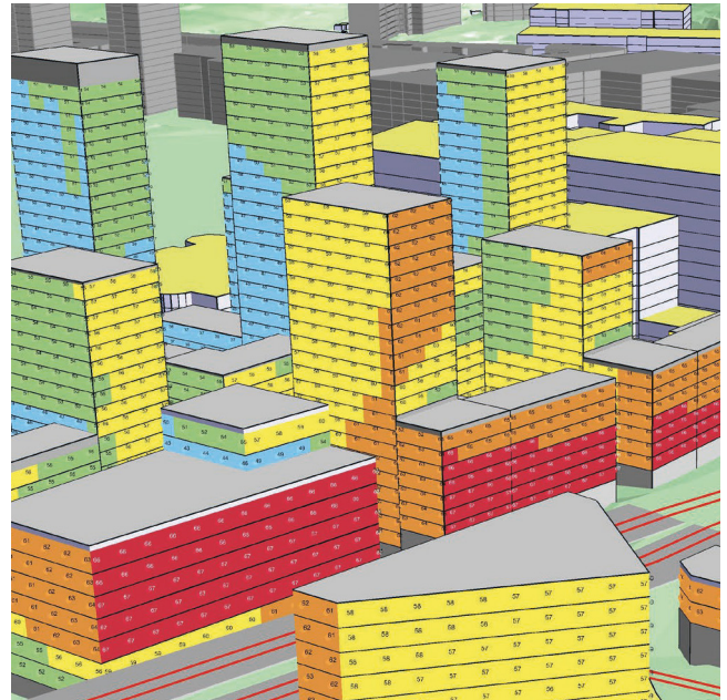
Exempel indragna högre byggnader mot Marievik med bullernivåer som högst 62 dB. Här krävs en medveten fördelning av lägenhetsstorlekar för att klara riktvärden. Bild Structor.
