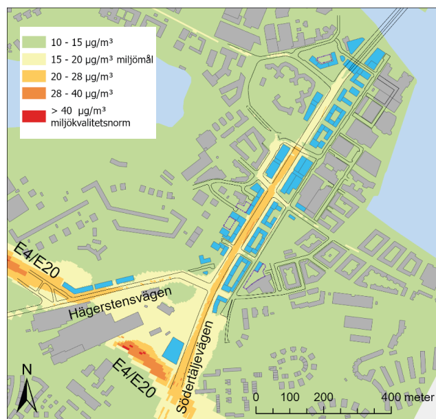
Beräknad årsmedelhalt av partiklar, PM10 ( \mu\text{g}/\text{m}^3 ) år 2040 efter genomfört planförslag längs Södertäljevägen. Halterna gäller 2 m ovan gatunivå för ett normalt meteorologiskt år. Inget överskridande av miljö kvalitetsnormen inom programområdet. Illustration SLB-Analys
