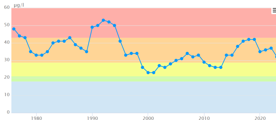
Figur 5. Totaltfosfor i Saltsjöns (del av Strömmen) ytvatten (treårsmedelvärden), augustivärden 1976–2023. Halterna visas mot bakgrund av intervall för statusklasser enligt HVMFS 2019:25. Målet för vattenarbetet, god status, är 22 µg/l (grönt fält). Diagram från Miljöbarometern Stockholm.
