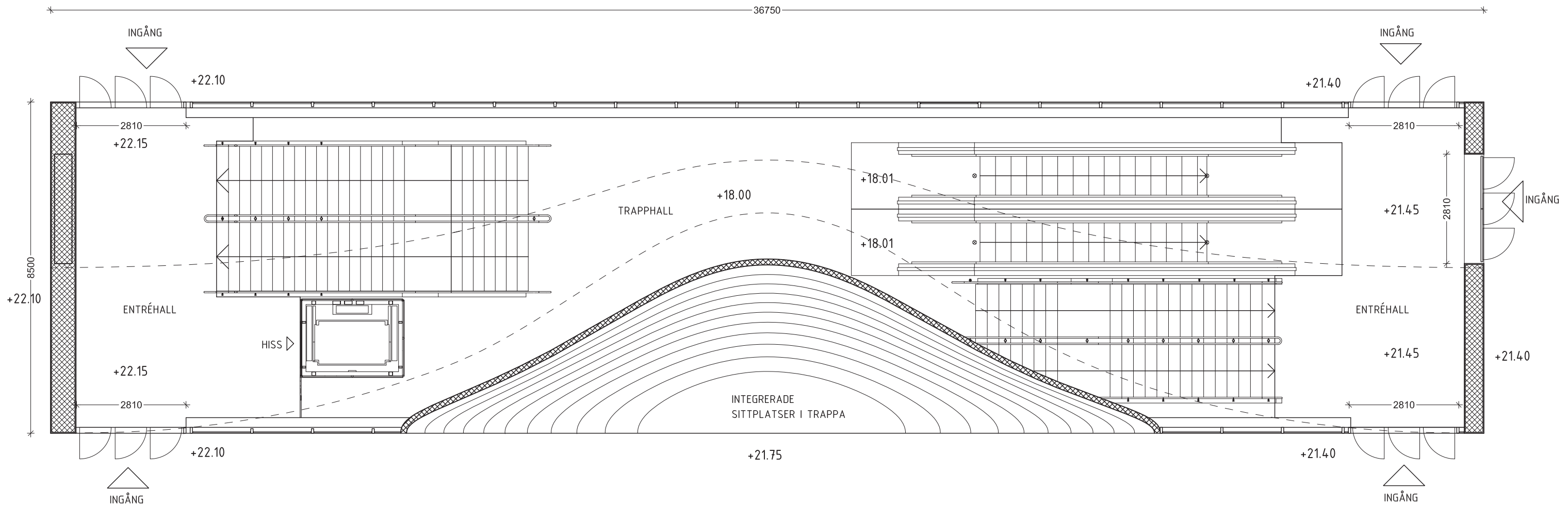
PLAN 1:100
