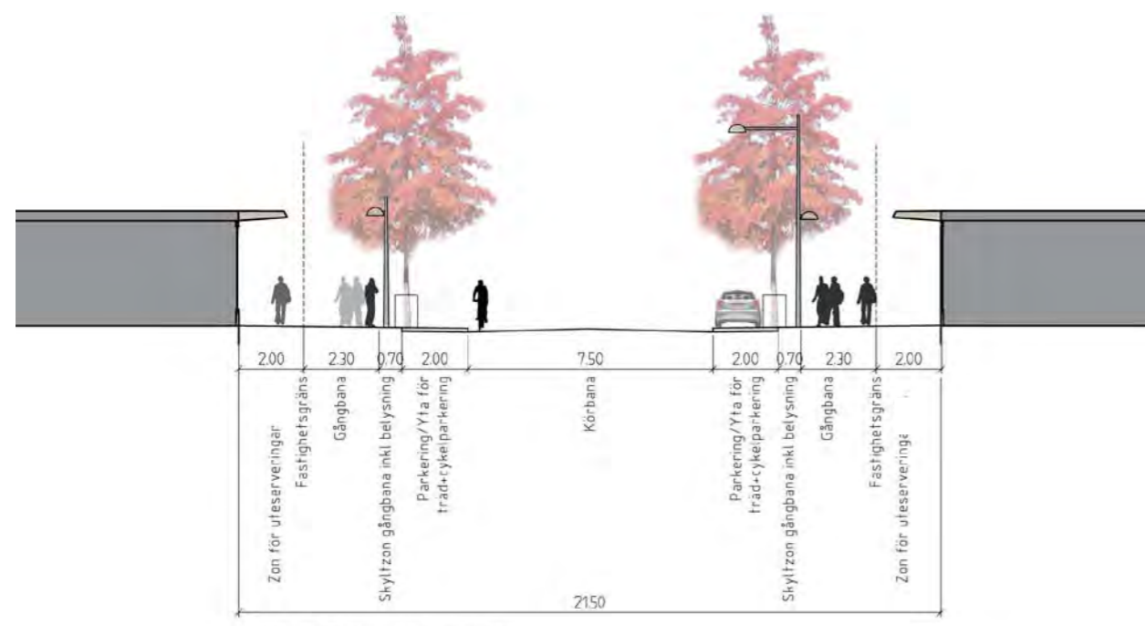
SEKTION SKALA 1:200
