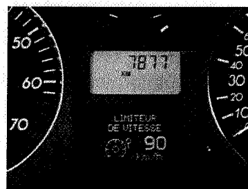
Fordonsintegrerad ISA (Renault prototyp)
