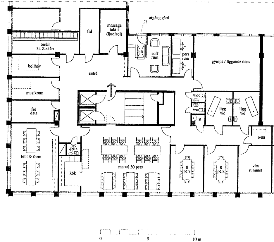
PLAN 1TR / 210 m 2
