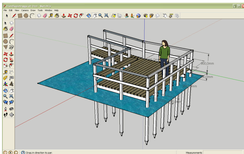
Bilaga 3. Kolardammarna, större bryggan. Observera att bryggan planeras byggas som flytbrygga.
