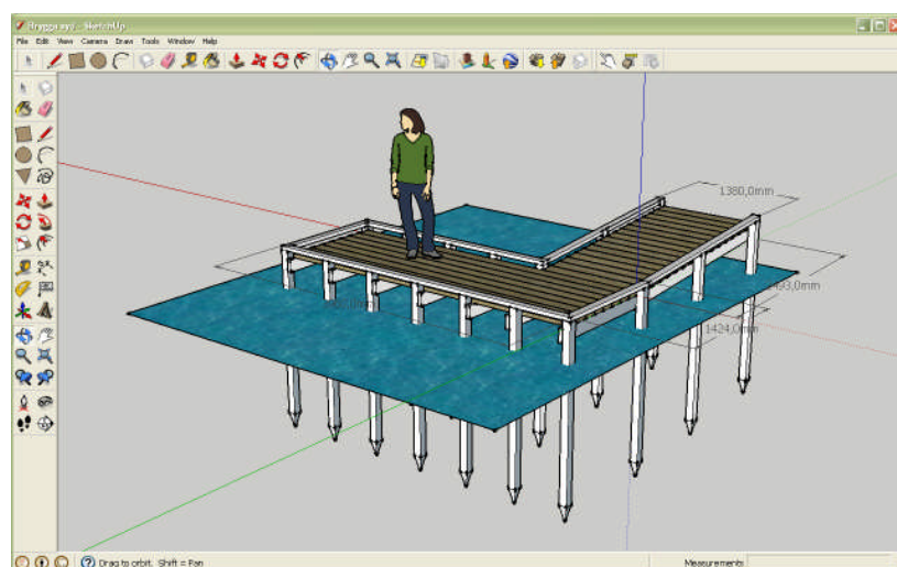
Bilaga 4. Kolardammarna, mindre brygga.
