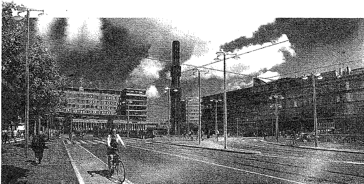
Illustration av förändrade belysnings- och kontaktledningsstolpar samt kontaktledning vid Sergels torg. Bildens visar även hur kontaktledningens bärlinor fästs i stolpar samordnat med belysningen
