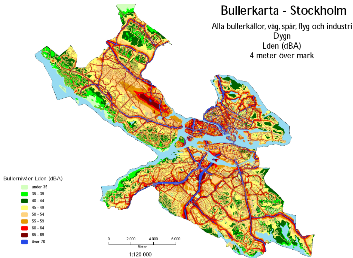
Figur 17 Bullerkarta - Stockholm
