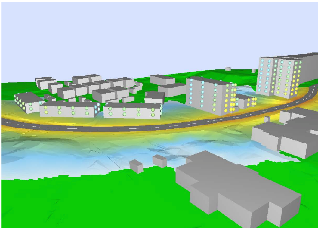
Figur 8. Tredimensionell återgivning av de beräknade ekvivalenta ljudnivåerna i nulägesituationen. Vy från söder.
