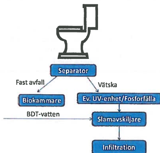
Figur 38. En flödesskiss över Aquatrons system. 117
