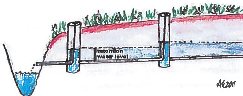
Figur 24. Principen för Reglerad dränering. Genom att minska utflödet från åkern minskar läckaget av växtnäringsämnen samtidigt som grödorna får en god vattentillgång. 76
