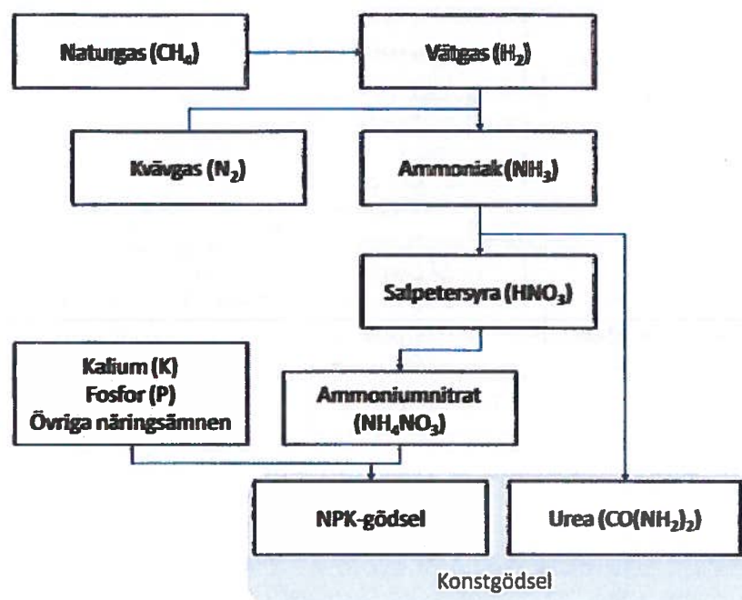
Figur 43. Tillverkningsprocessen för kvävegödsel.
