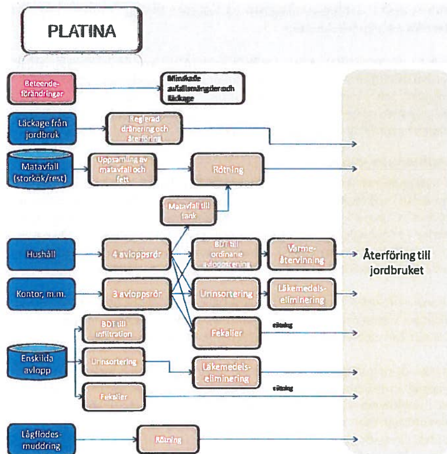
Figur 42. Exempel på teknik som kan uppnå Platina-nivå.
