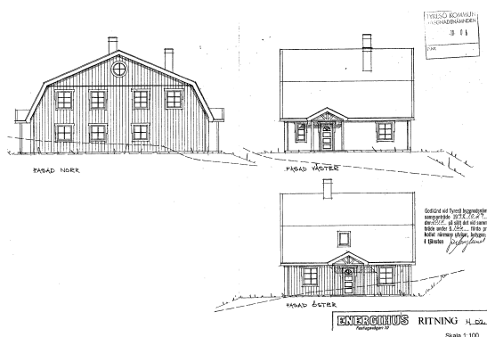
Bygglovritningar från 1998.
