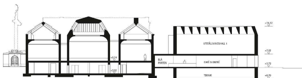
Sektion D-D
