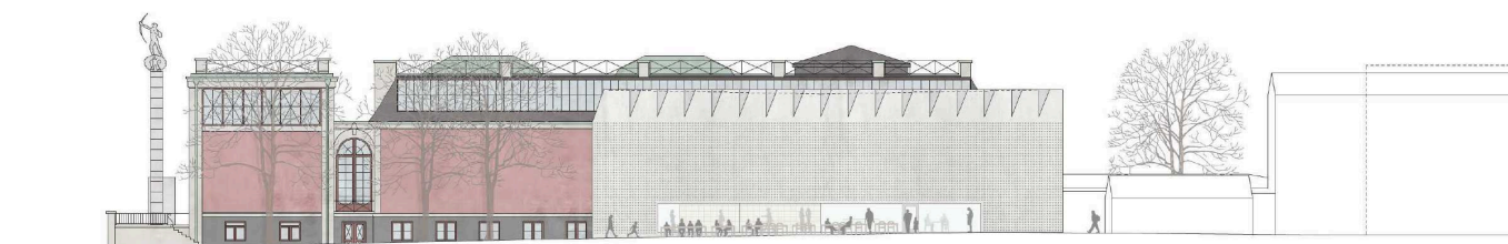
Västfasad. Bilden visar tävlingsförslagets 34-metersbyggnad. Bild: Wingårdhs
