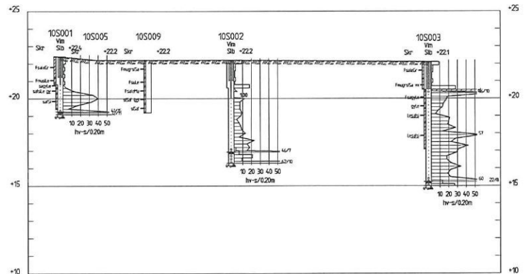
SEKTION A-A 1:100
