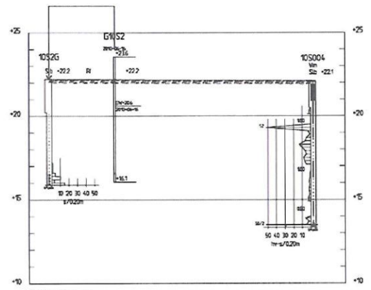
SEKTION B-B 1:100
