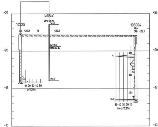
SEKTION B-B 1:100
