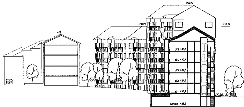
Sektion BB
