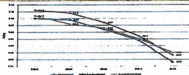
PISA - Resultatutvecklingen 2000-2012
