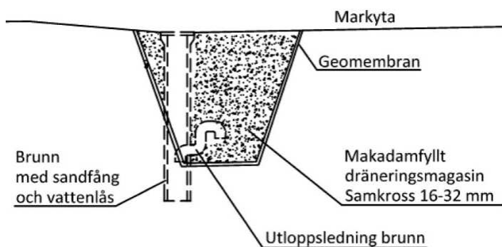
Principskiss för ett makadamdike
