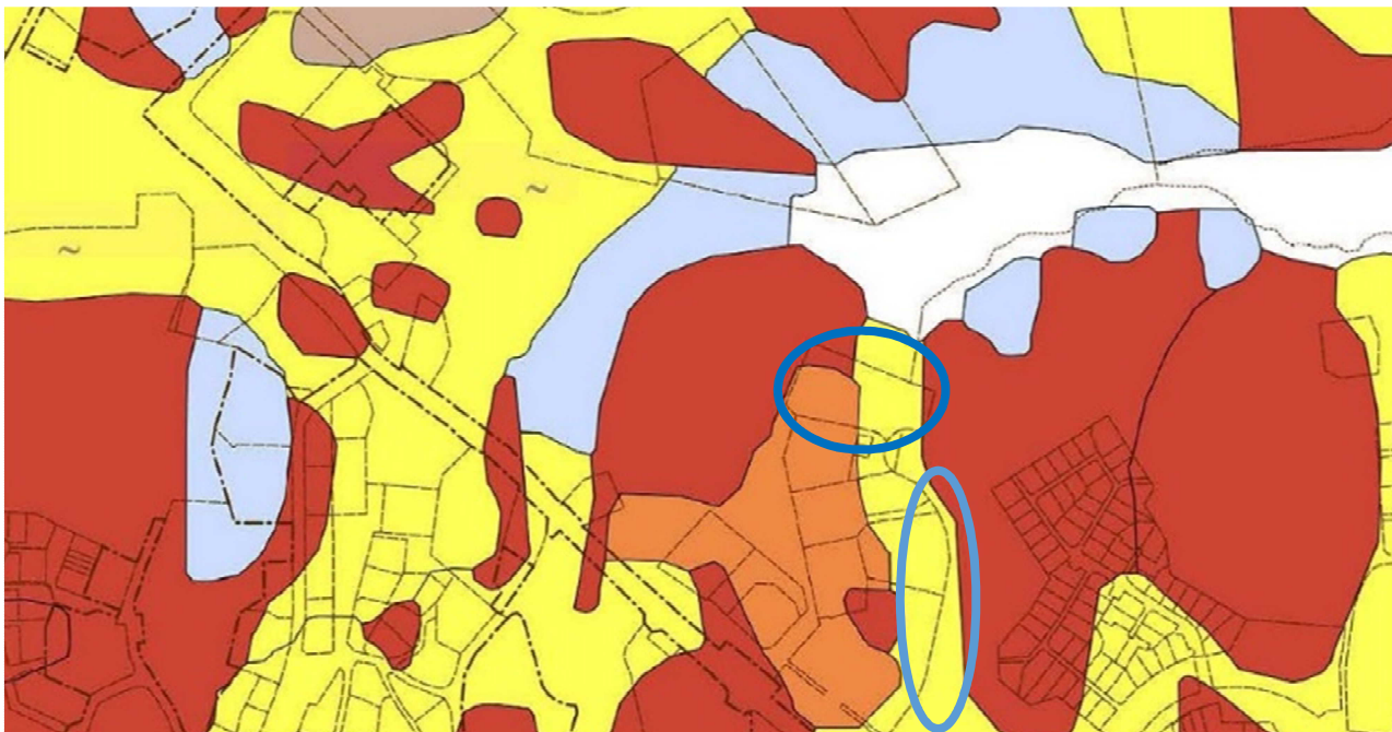
Karta 6 SGU:s jordartskarta. Gult markerar glacial lera, rött urberg och orange svallsediment grus. Blå ring markerar bebyggelseområdet och ny GC-väg.
