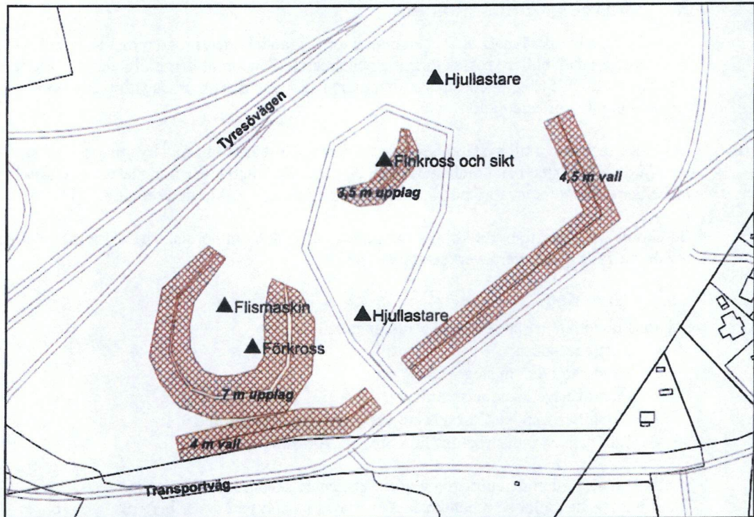
Figur 4. Bullerkällor och avskärmingar
