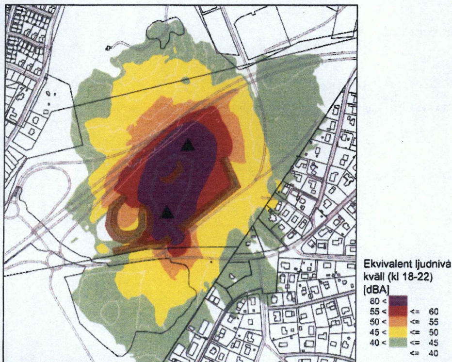
Figur 6. Ekvivalent ljudnivå, typisk verksamhet kvällsperioden, riktvärde 45 dBA. Se även bilaga 5.
