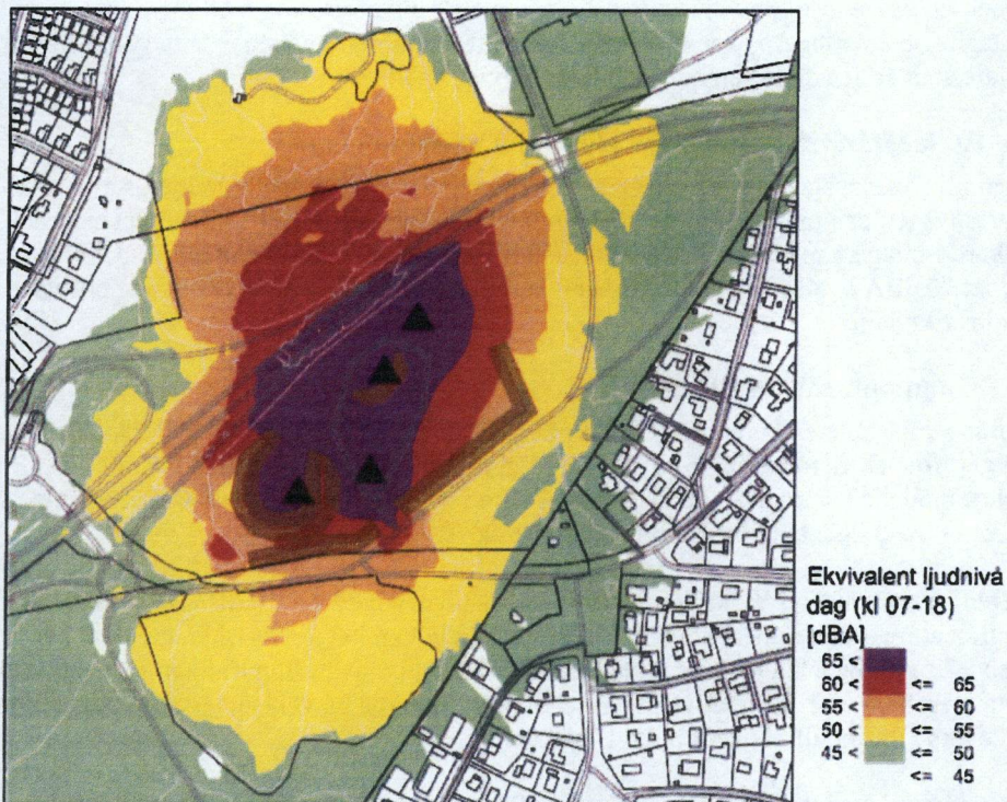
Figur 5. Ekvivalent ljudnivå, typisk verksamhet dagperioden, riktvärde 50 dBA. Se även bilaga 4
