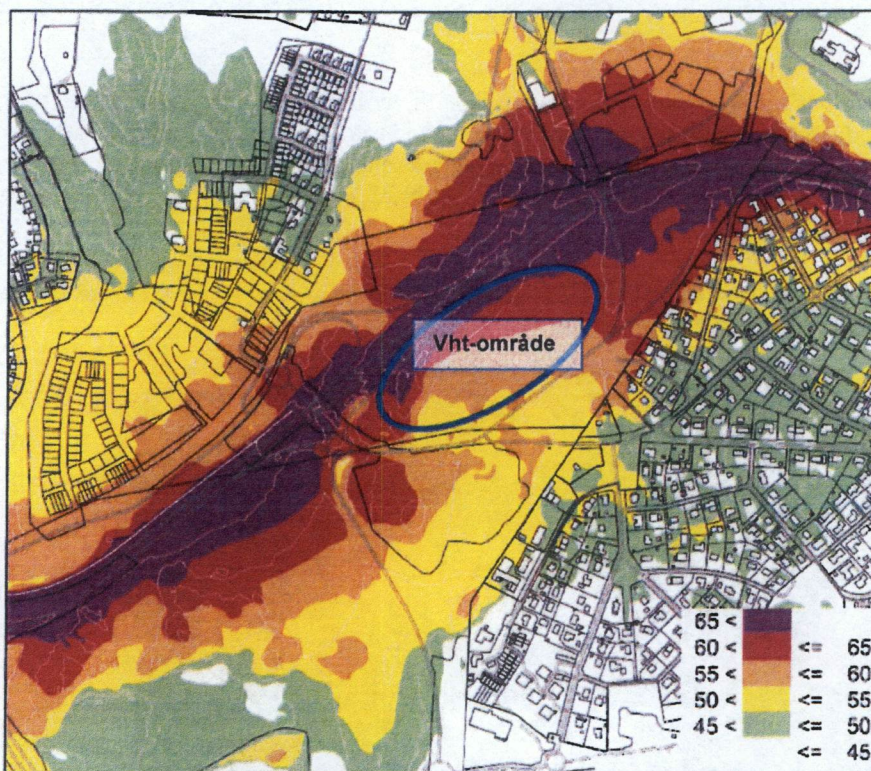
Figur 2. Trafikbuller, dygnsekvivalent ljudnivå (dBA), från Tyresövägen.
