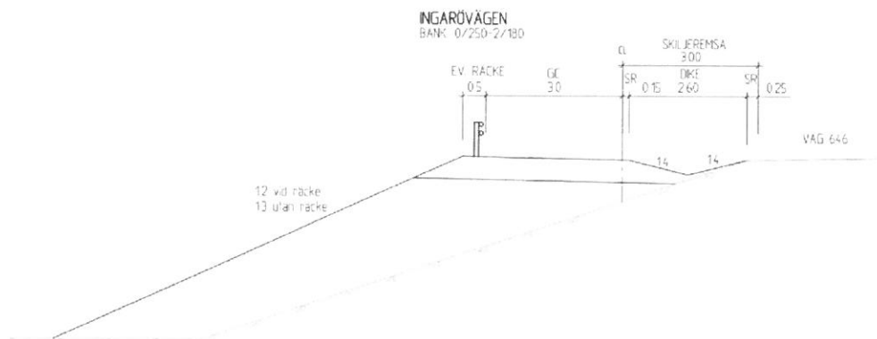
Figur 20. Skärning. Gång- och cykelväg med skiljeremsa mellan väg 646 och gång- och cykelväg
