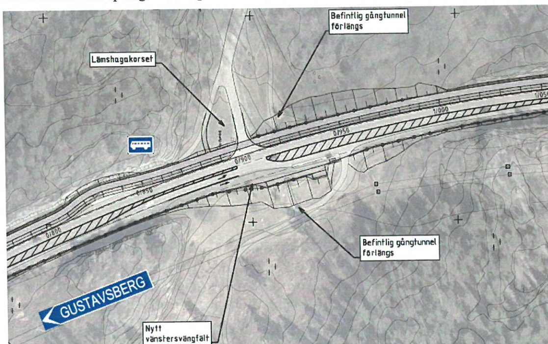
Figur 2 Infarten till Lemshaga. Utdrag ur Gustavsberg_samradshandling_illustrationsplan_02
