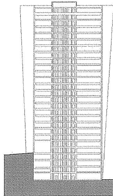
Sektion D-D
