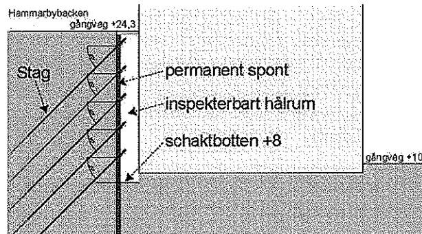
Enkel principskiss över konstruktion längs Hammarbybacken
