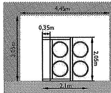
Skärning genom befintliga rör med fjärrvärme. Ny skatehall kan byggas över och runt ledningarna.
