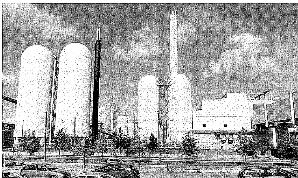
Figur 11. Bild på Hammarbyverket från tomten där gasblandningsstationen är placerad. Ackumulatortankarna ses närmst Hammarby Allé.
