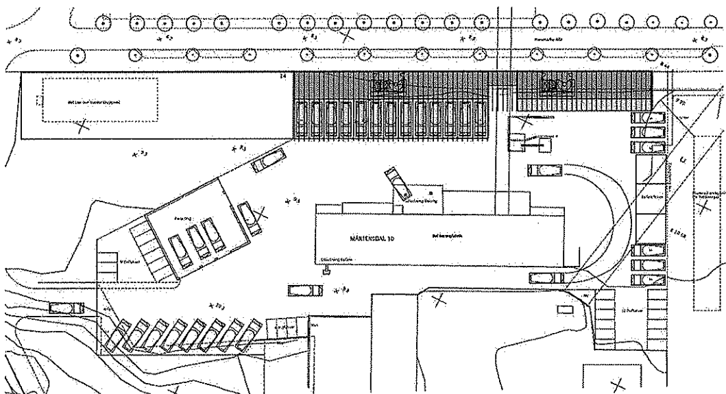
Figur 7. Illustrationsplan över nya kontorshuset på Mårtensdal 10.
