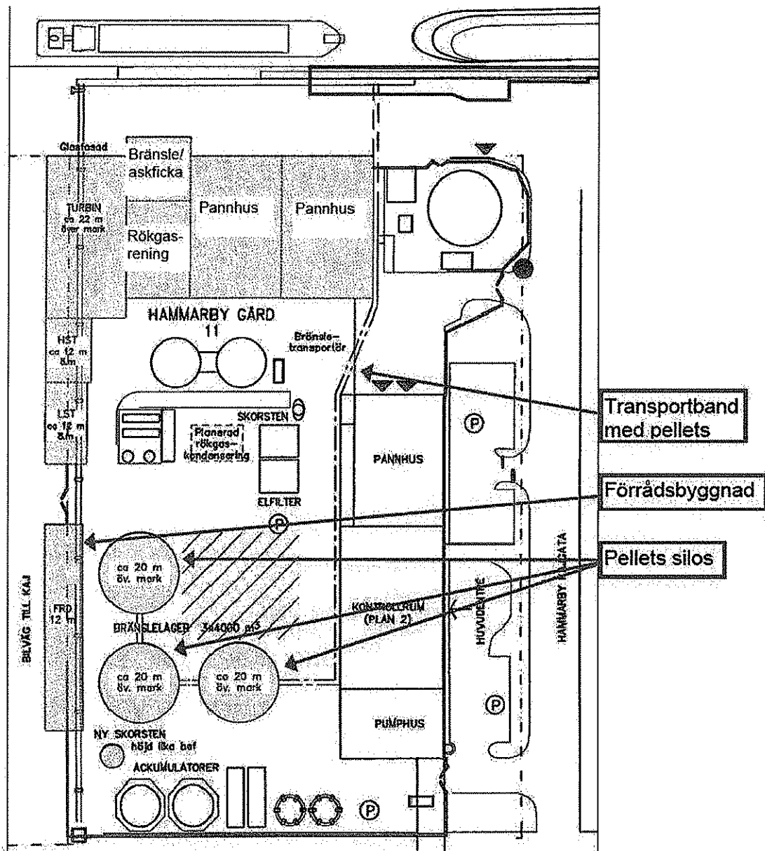
Figur 12. Principskiss över Fortum Värme's befintliga delar samt planerade utveckling av Hammarbyverket inom Hammarby Gård 11 med Hammarbykanalen i norr. Gula byggnader redovisar tillkommen bebyggelse. Skiss tagen från Swecos riskanalys [2]. Utökningen med pellets silos är numera ej aktuellt.
