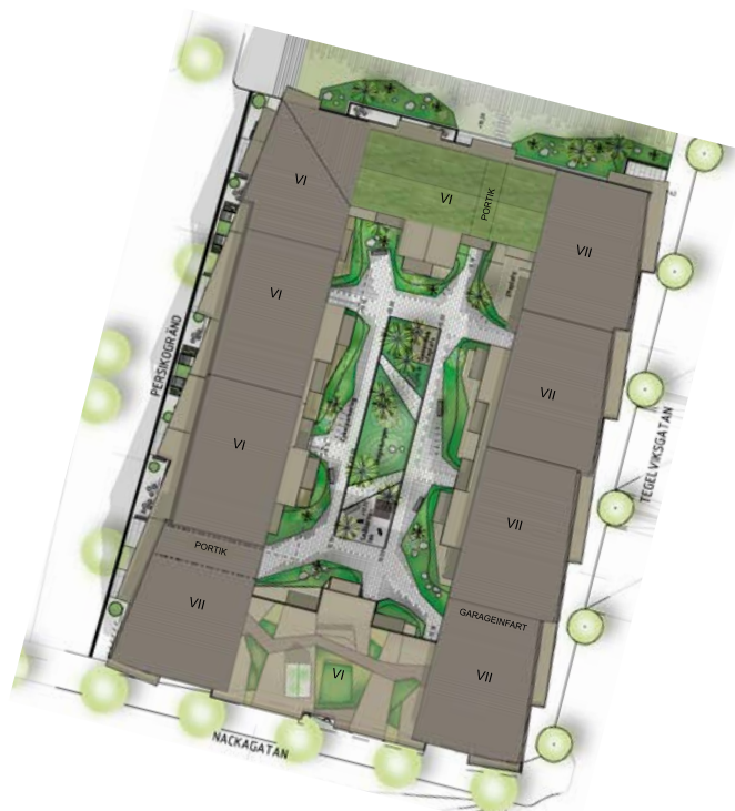
Planutsnitt 1:1000
