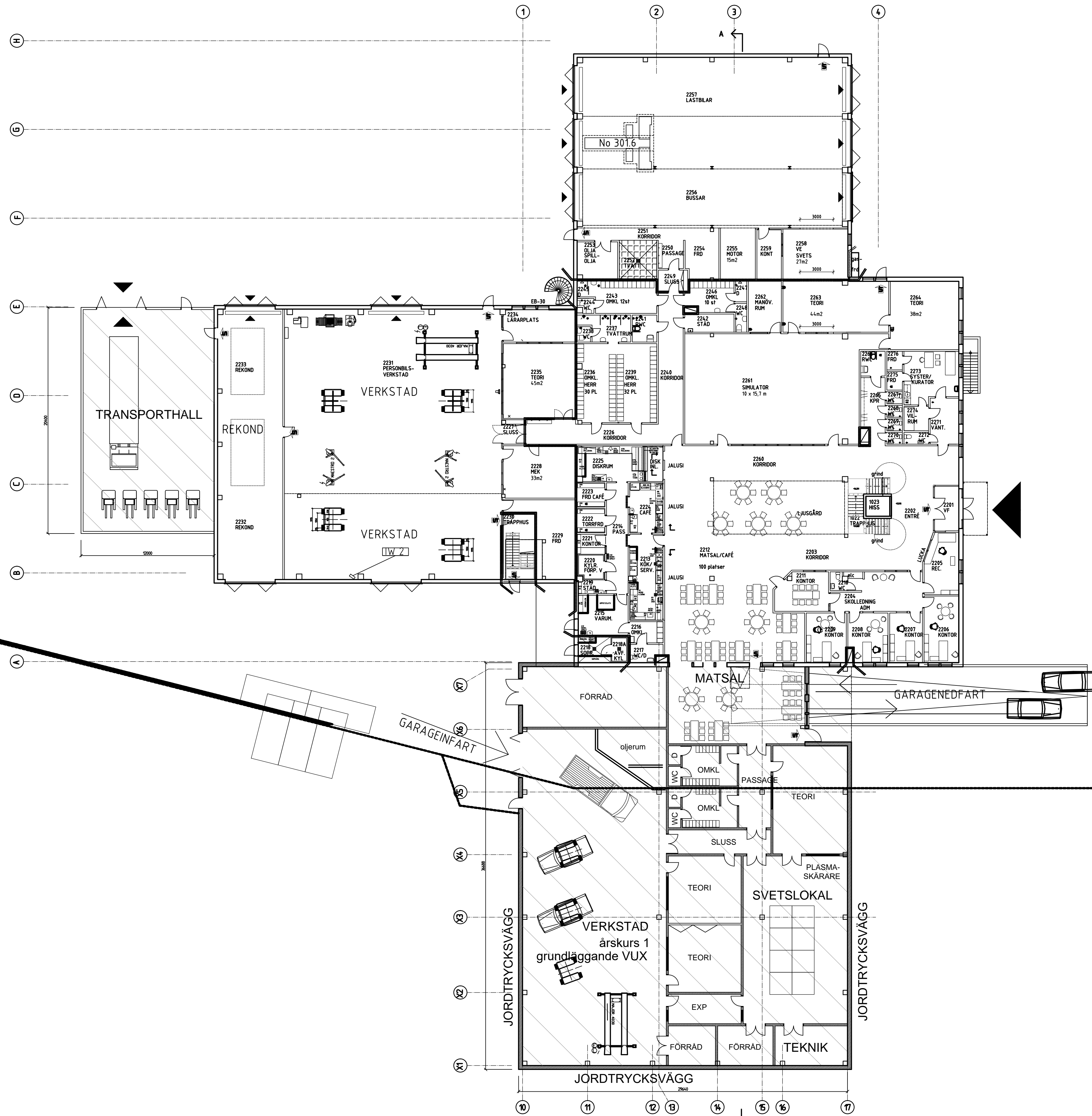
PLAN 1 tillkommande yta: 1090m 2 + 245m 2 (Byggnadsarea)
