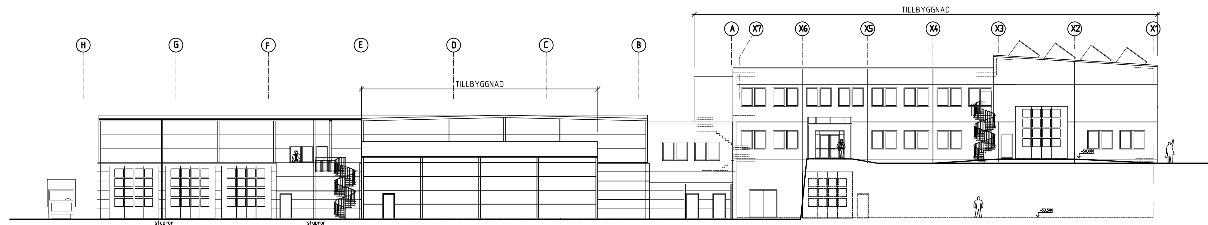
fasad mot väster
