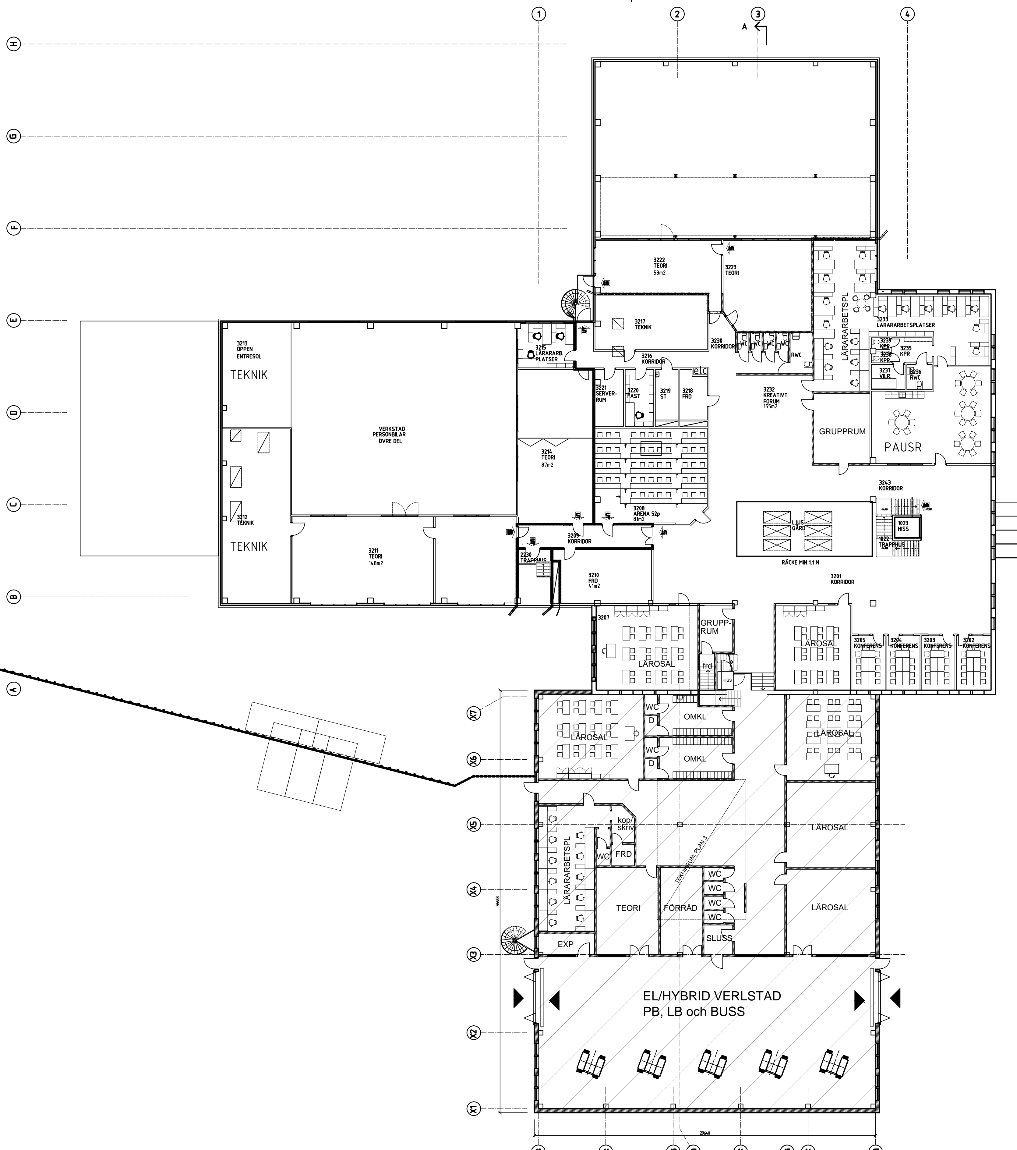
PLAN 2 tillkommande yta: 1090m2 (Bruttoarea)
