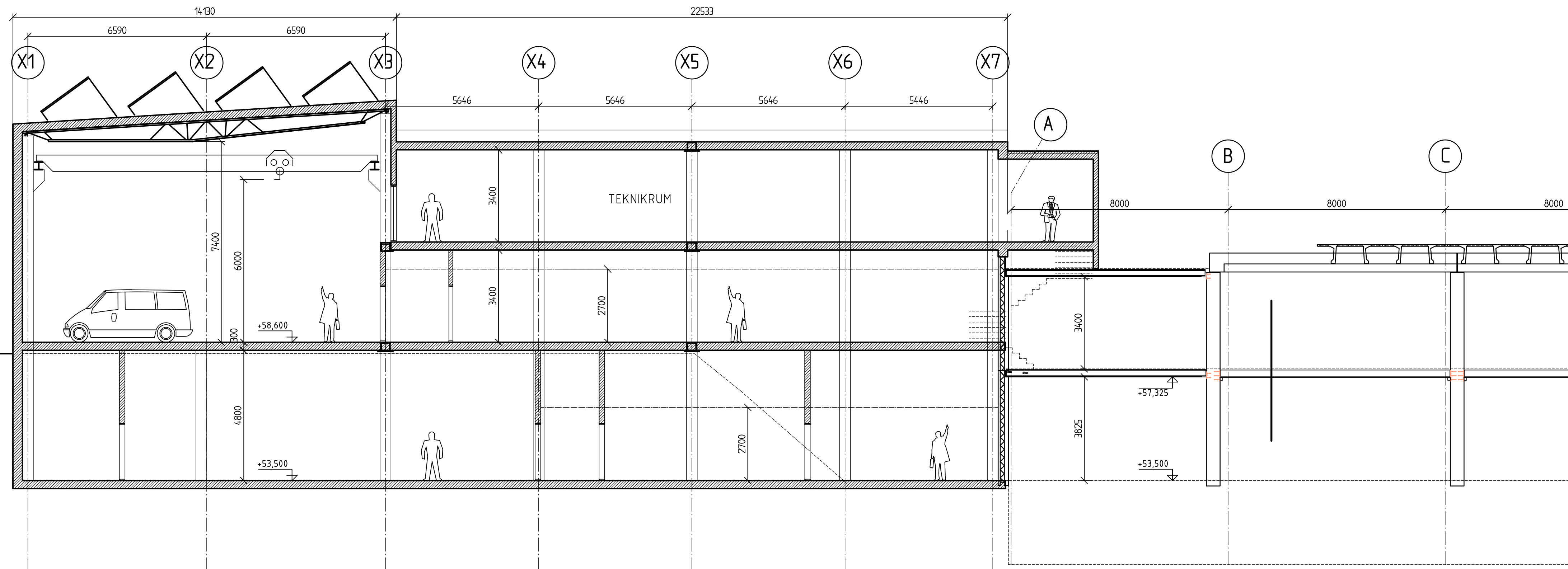
sektion A-A
