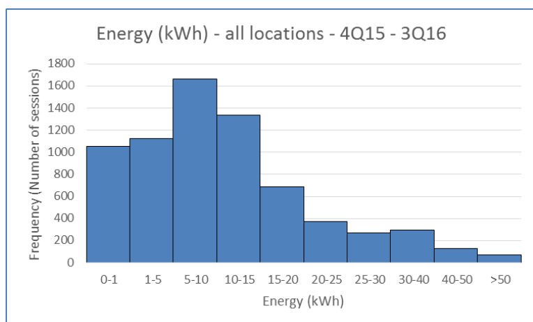
Figur 5. Histogram som visar överförd energi för snabbbladdare för perioden aggregerat resultat för alla snabbbladdplatser.
