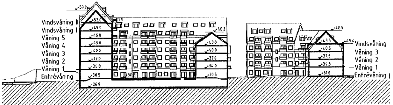
Sektion 3 genom kvarter C och D (Källa: Sandellsandberg)
