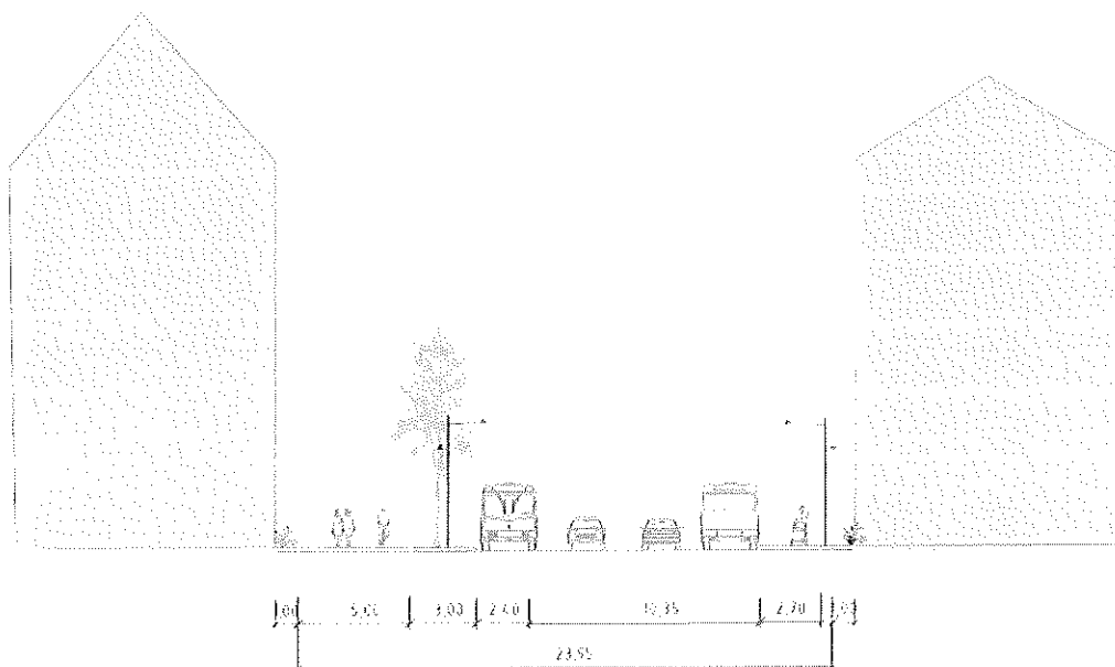
Typsektion i skala 1:200 - Grycksbovägen (Källa: Sweco Architects AB)
