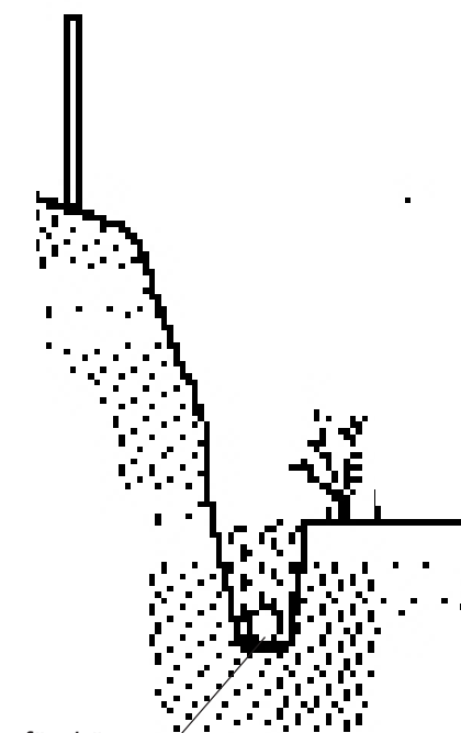
Täckdike för dränering av avrinning från berget
