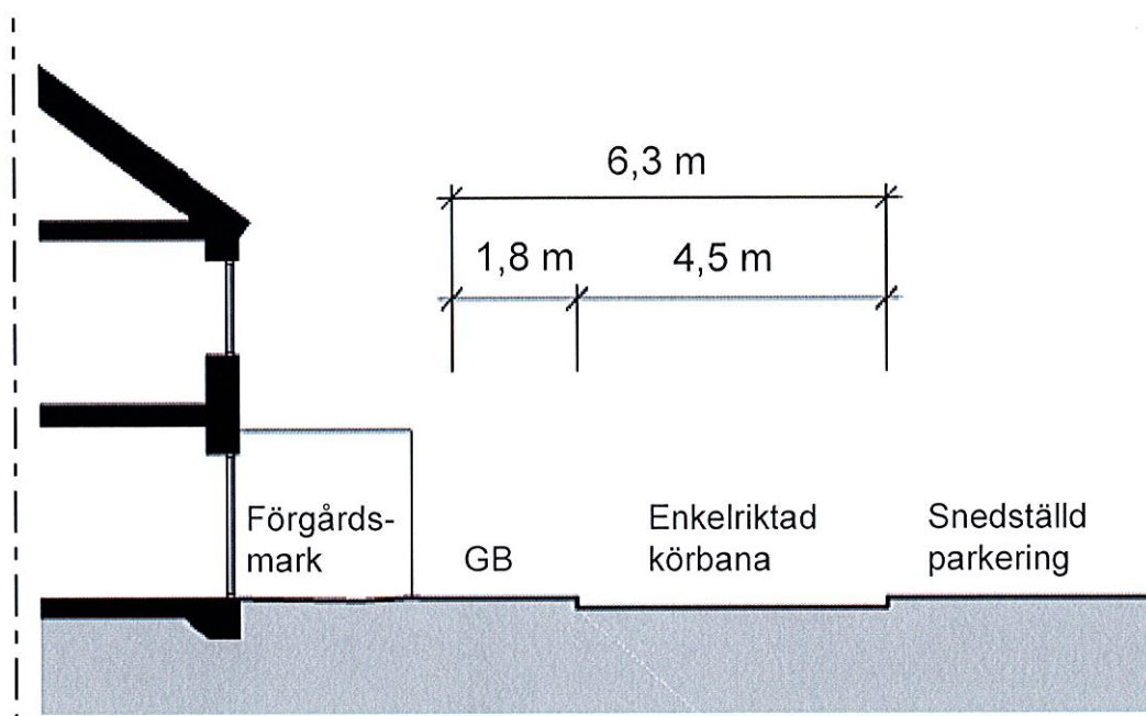
Sektion B-B
