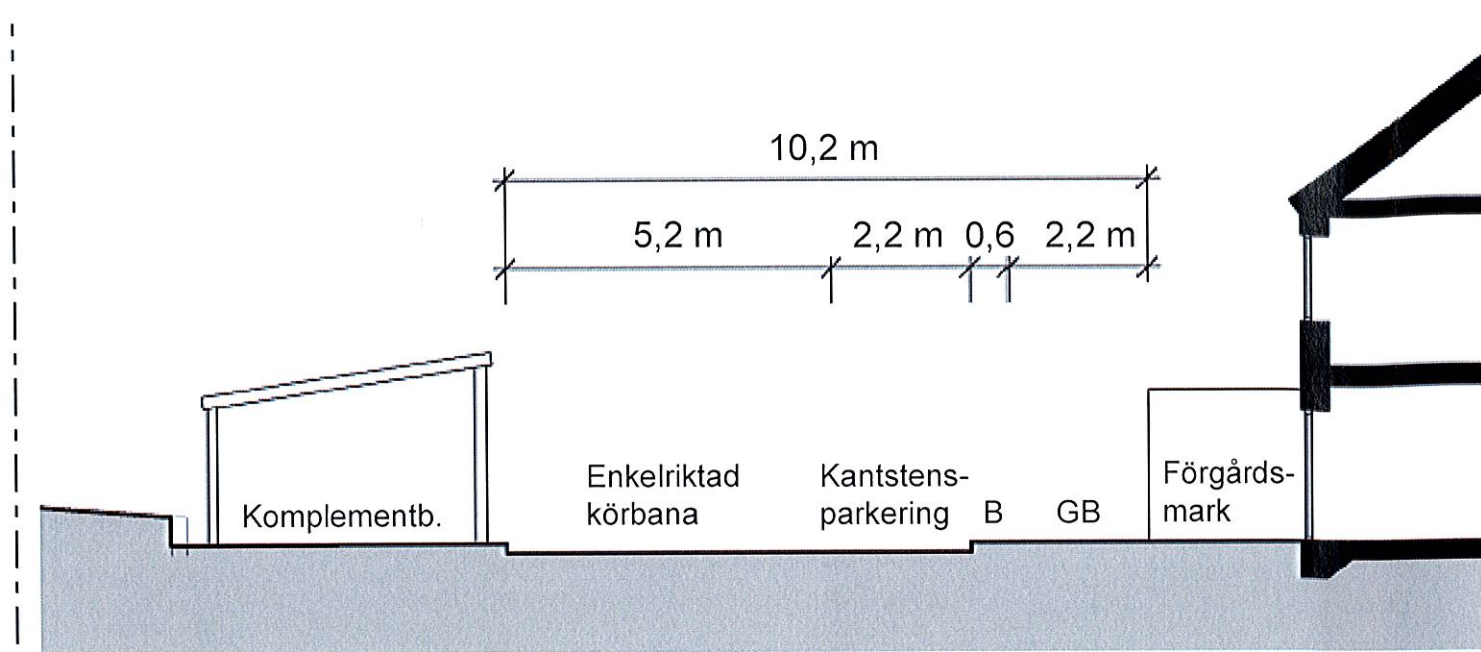
Sektion A-A
