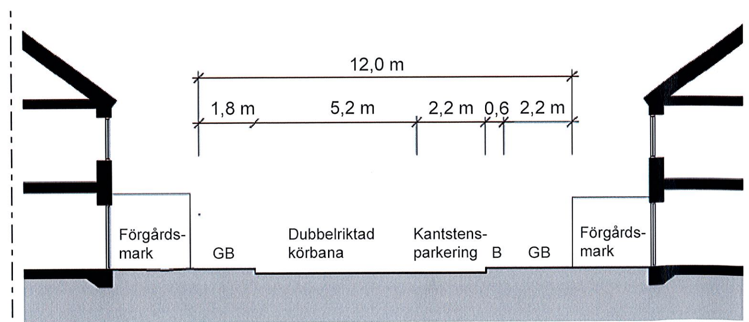
Sektion C-C
