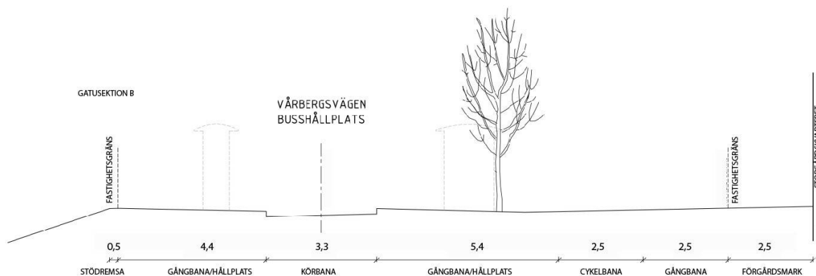
Gatusektion A samt gatusektion B, vilka visar planerad ombyggnad av Vårbergsvägen. Måttangivelser i meter.
