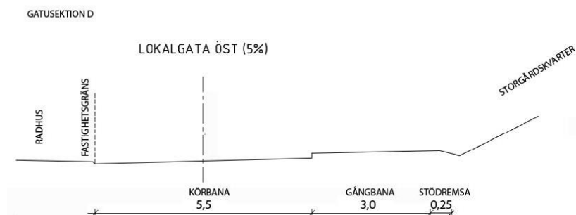
Gatusektion C och gatusektion D, vilka visar nya lokalgator. Måttangivelser i meter. Procentantal anger gatans lutning.
