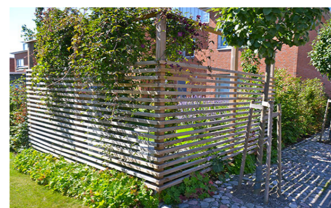
Exempel spaljéstaket
