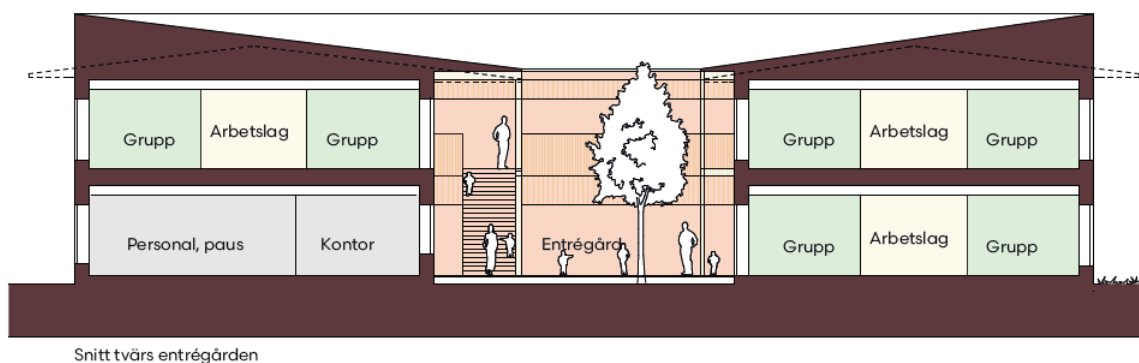
Snitt tvärs entrégården
