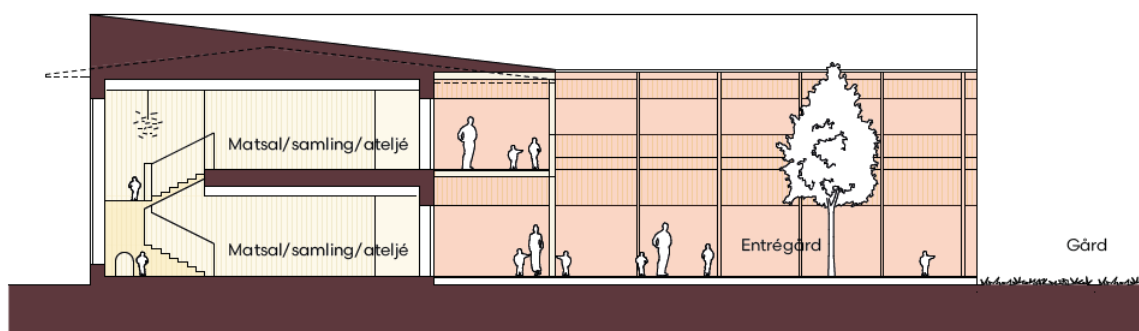
Snitt längs entrégården
