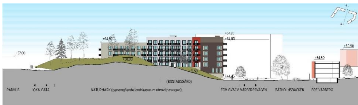
TVÄRSEKTION A-A
