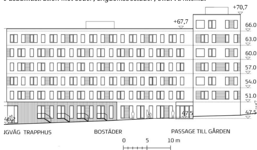
Fasadillustration mot öster (mot Vårbergsvägen), ungdomsbostäder, bild: Arkitema.
