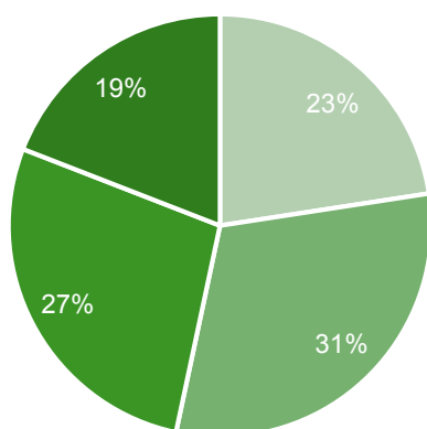
Figur 7. Bedömning av ljusförhållandena för enskilda jätteeekar, andelen av totalt 2 703 ekar år 2006 och 2 701 ekar år 2017.
