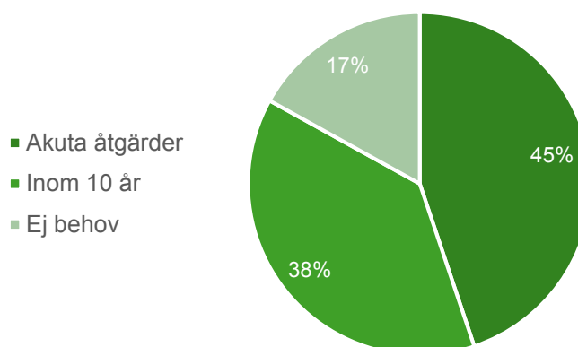
Figur 27. Tidsaspekt för restaureringsbehov av ekområden, andelen av totalt 918 områden år 2006 och 885 områden år 2017.
