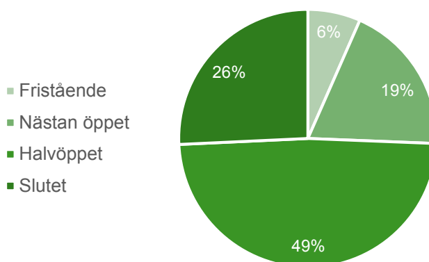
Figur 7. Bedömning av ljusförhållandena för enskilda jätteeekar, andelen av totalt 2 703 ekar år 2006 och 2 701 ekar år 2017.
